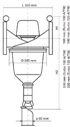
Filtre Cillit Turbo Automatique
