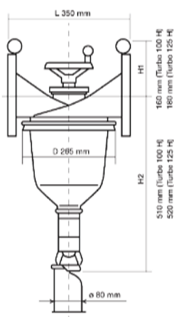
Filtre Cillit Turbo Manuel
