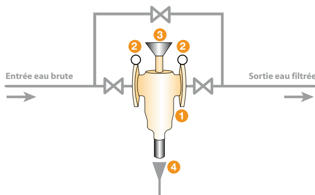
Filtre Cillit Turbo Automatique
